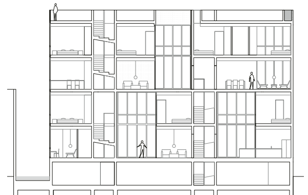
Schnitt B
